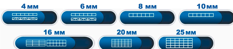
Рисунок 19. Типы структур сотового поликарбоната.
