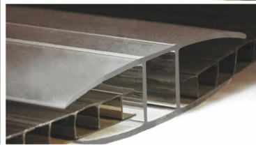
HP - профиль СОЕДИНИТЕЛЬНЫЙ НЕРАЗЪЁМНЫЙ
