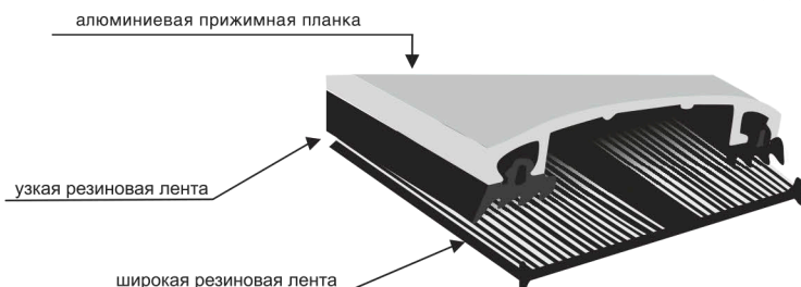
Рисунок 14а. Металлические соединительные профили.
