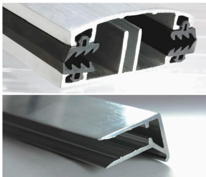
Рисунок 14а. Металлические соединительные профили.
